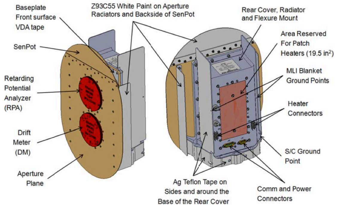
Fig. 9 ICON Ion Velocity Meter (IVM)
